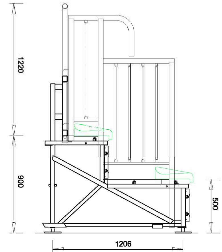
VISTA LATERALE NUOVE TRIBUNE FISSE SCALA 1:200
