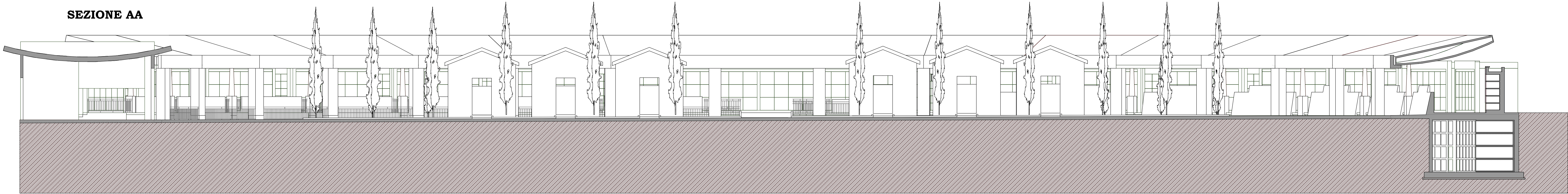
SEZIONE BB
