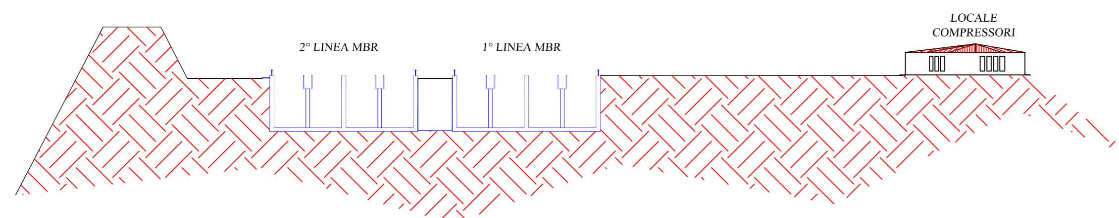
SEZIONE A-A
