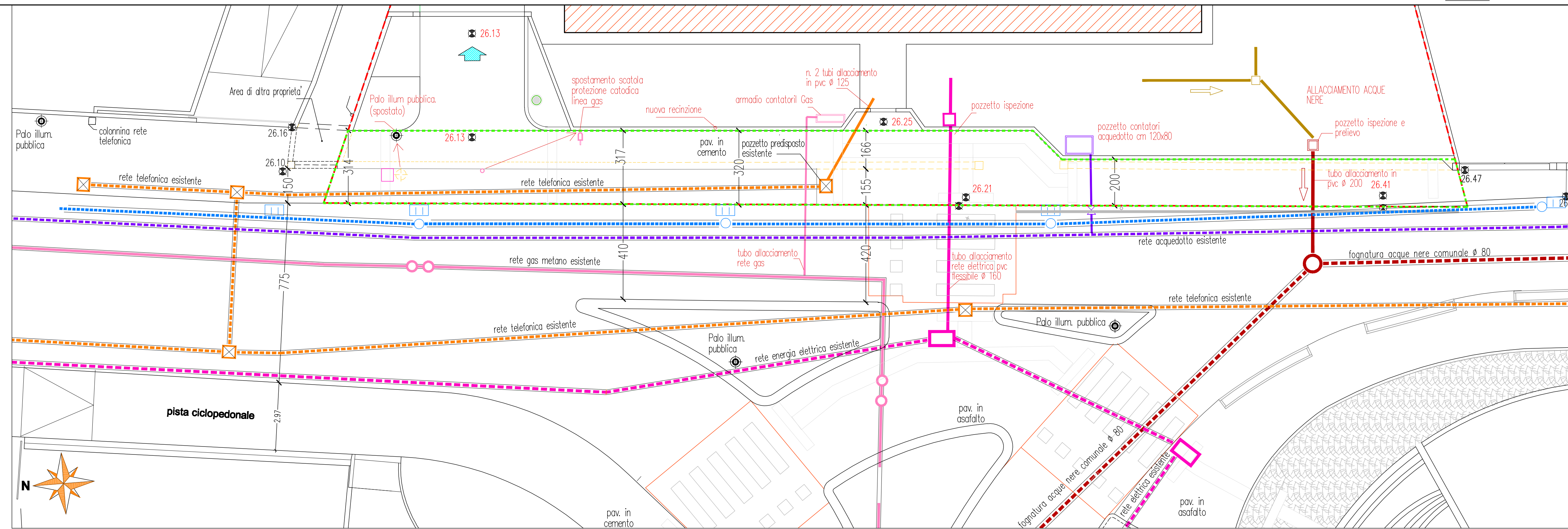
Planimetrie allacciamenti reti tecnologiche 1:100
