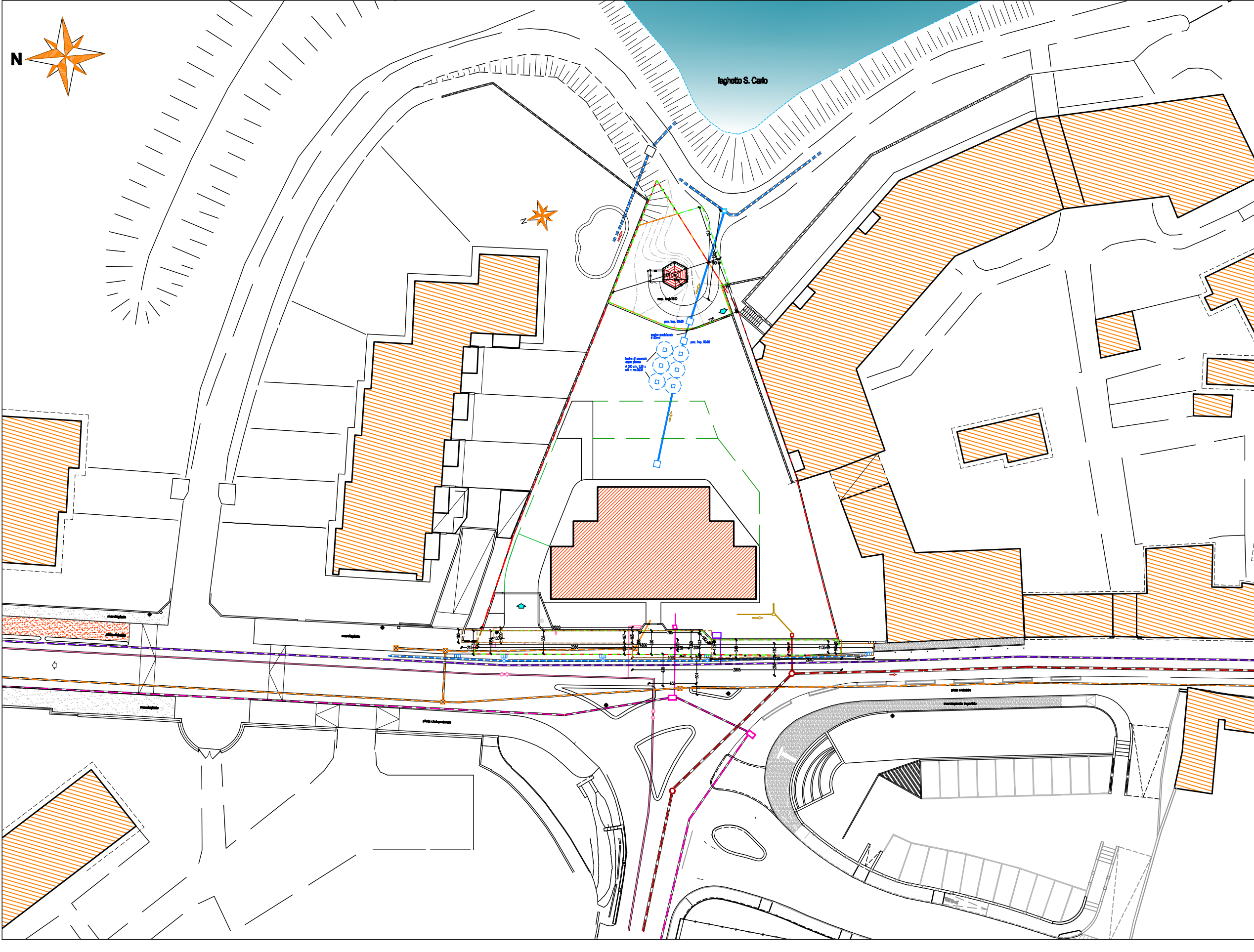
Planimetria generale 1:500
