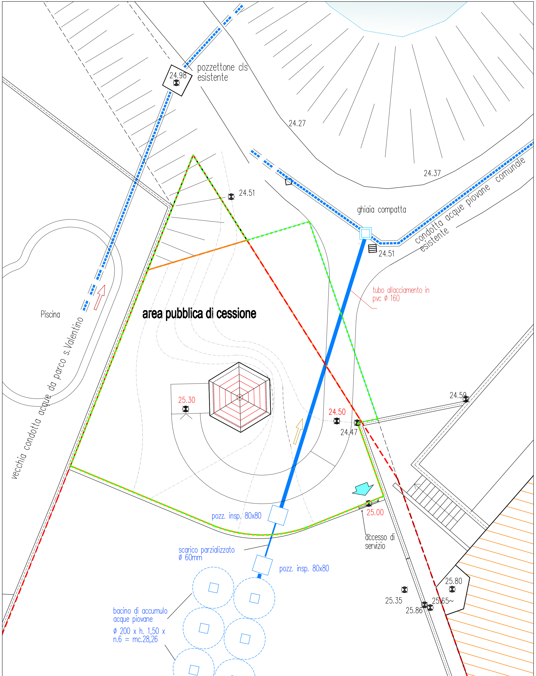
Planimetrie allacciamenti reti tecnologiche 1:100
