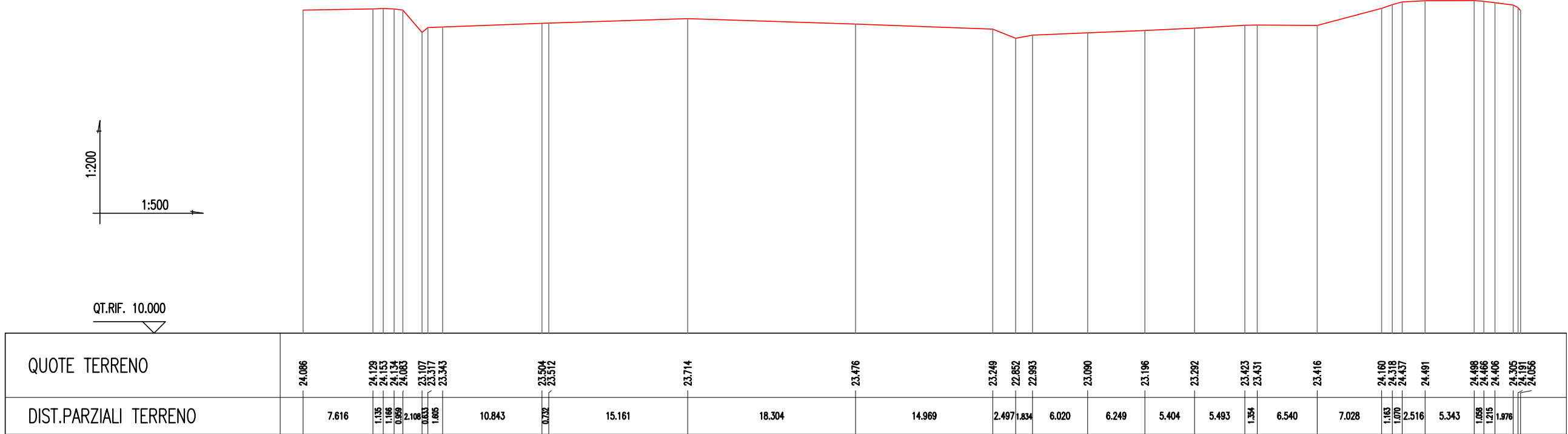
SEZIONE B
