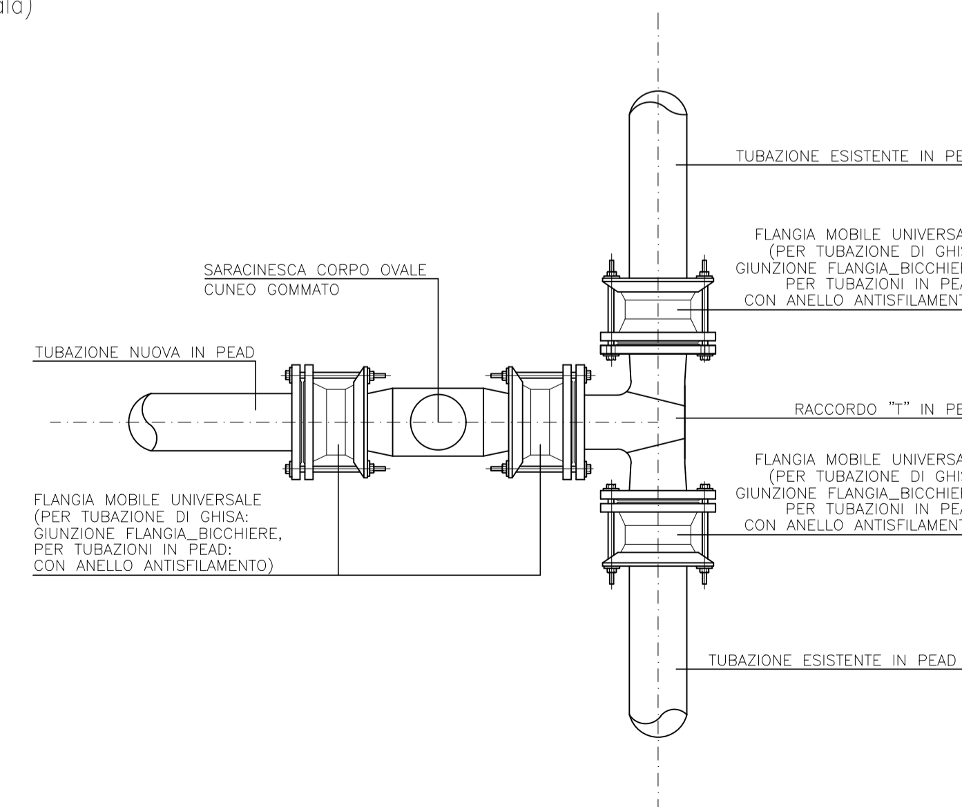
PARTICOLARE INTERCETTAZIONE LINEA PRICIPALE (non in scala)
