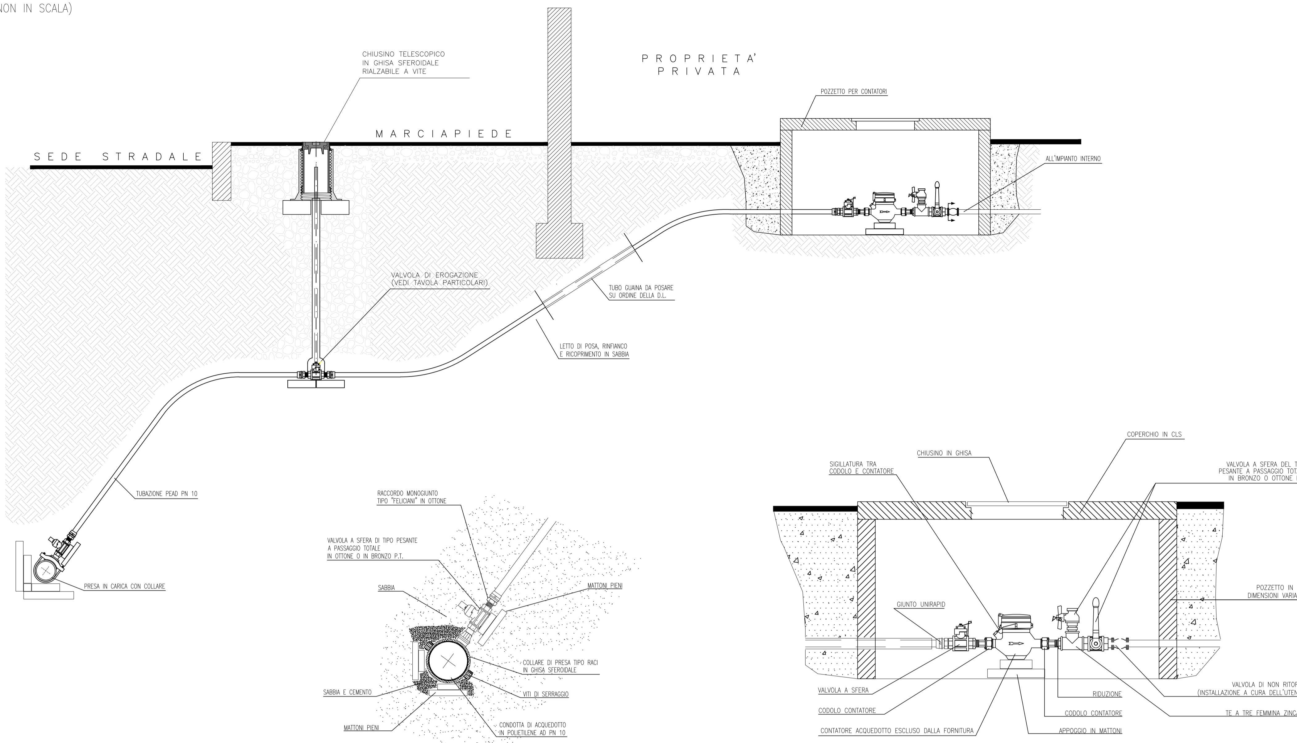
PARTICOLARE POZZETTO CONTATORI (NON IN SCALA)
