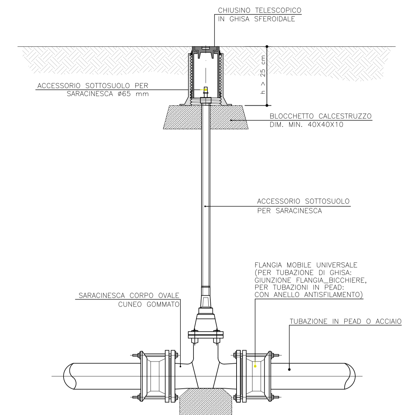
PARTICOLARE SARACINESCA IN LINEA. (non in scala)
