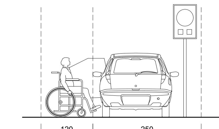
PARTICOLARE PARCHEGGI - 1:50
