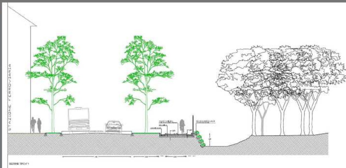
Sezione Tipo
